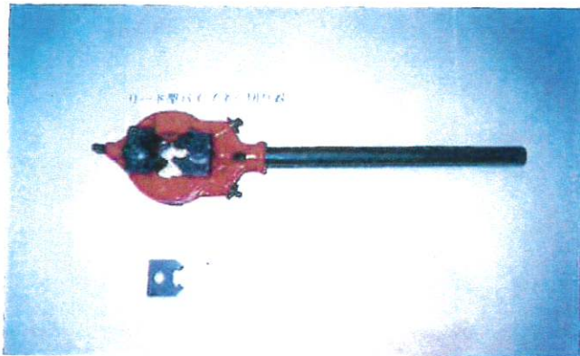
◎オスタ型パイプねじ切り機 ○
